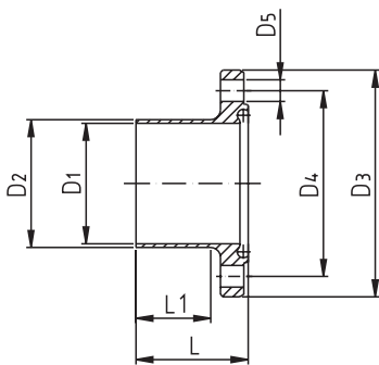
Nutflansch DIN nut flange DIN
