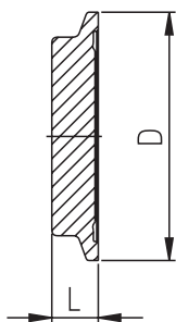
Blind-Bundklemmstutzen Zoll blind clamp
