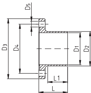
Bundflansch DIN liner flange DIN
