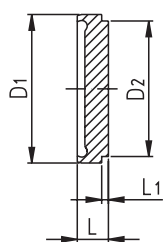
Blindbundstutzen ISO liner blank ISO
