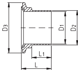
Nutklemmstutzen ISO clamp nut ISO
